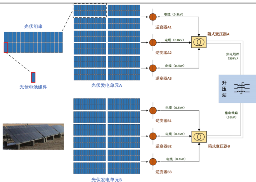
图 2.2-1 光伏场区示意图
