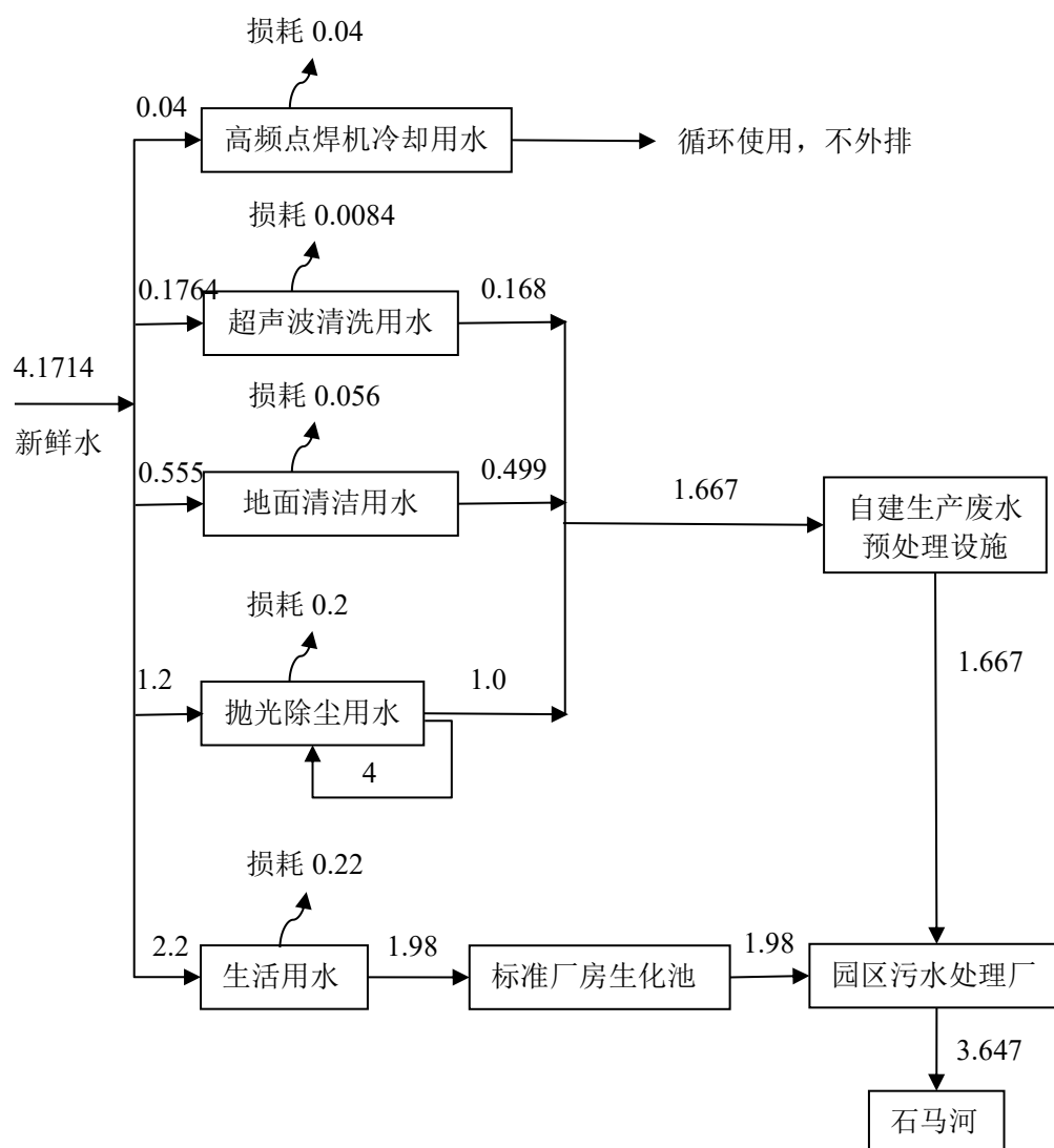
图 2.7-1 最大水平衡图 单位: m³/d
